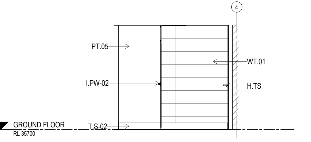
E ELEVATION UNISEX C/R.04 Scale: 1: 50
