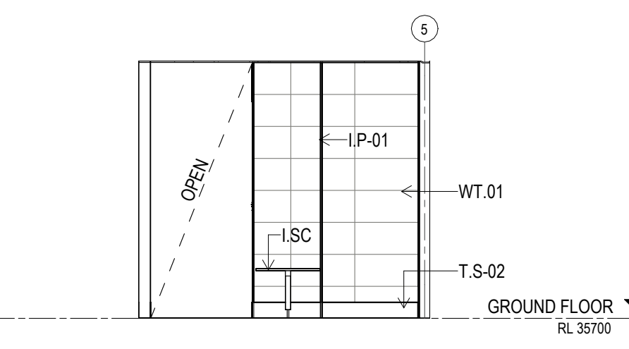
L ELEVATION UNISEX C/R.03 Scale: 1: 50
