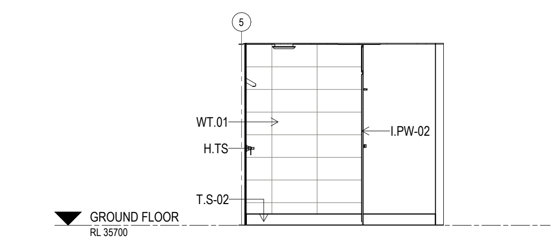
K ELEVATION UNISEX C/R.03 Scale: 1: 50
