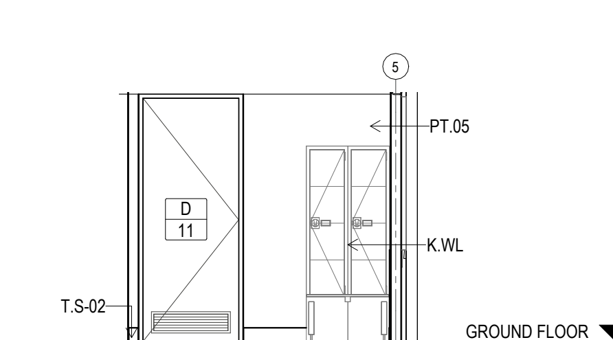
J ELEVATION UNISEX C/R.03 Scale: 1: 50
