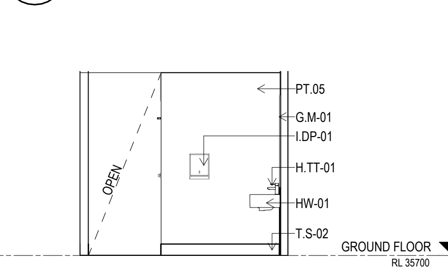
D ELEVATION UNISEX C/R.04 Scale: 1: 50
