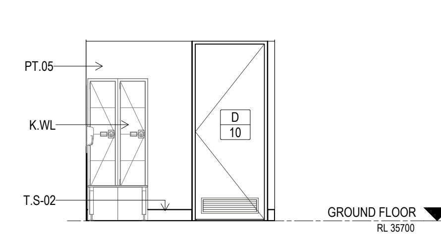
B ELEVATION UNISEX C/R.04 Scale: 1: 50
