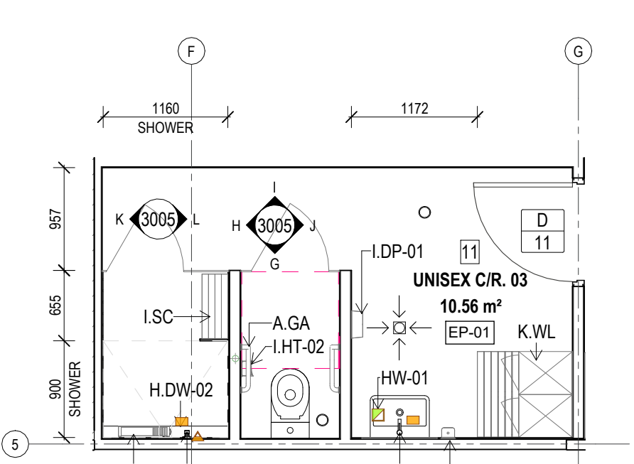
3 PLAN UNISEX C/R.03 Scale: 1: 50
