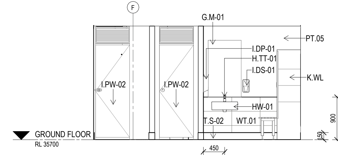
A ELEVATION UNISEX C/R.04 Scale: 1: 50
