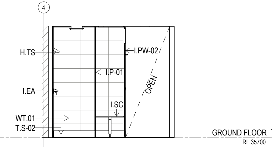
F ELEVATION UNISEX C/R.04 Scale: 1: 50
