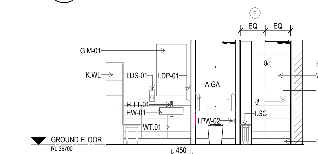
G ELEVATION UNISEX C/R.03 Scale: 1: 50
