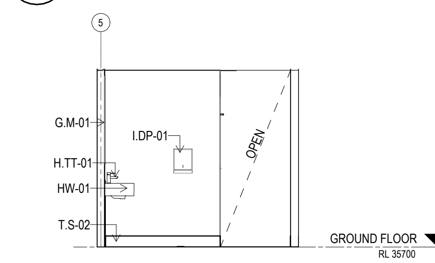
H ELEVATION UNISEX C/R.03 Scale: 1: 50
